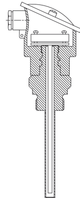
Со вставкой DIN 43762
