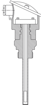
С установленным внутри кабельным датчиком
